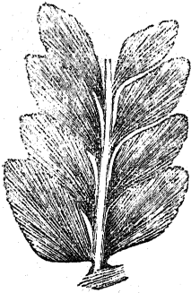
चित्र १२ बहुपत्रक या फर्न
